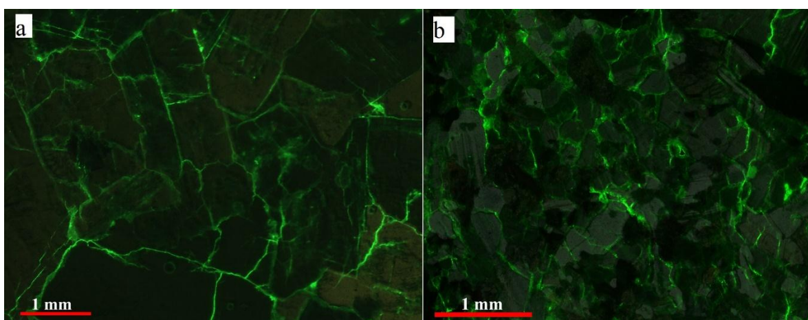
شکل ۸. تصاویر مقطع نازک سنگ دیوریت و گرانیت در زیر نور فلورسانس در آستانه CI؛ (a) گرانیت (b) دیوریت.
