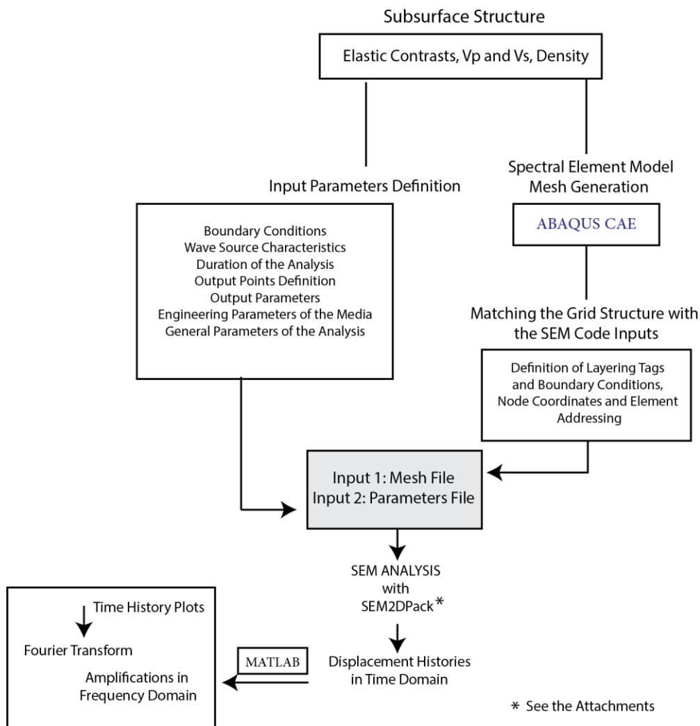
شکل ۳- فلوچارت تهیه ورودی‌های اولیه، مدل‌سازی عددی و تهیه خروجی‌ها.
