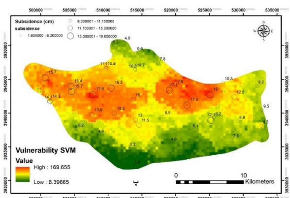
شکل ۵. الف) نقشه فرونشست ماهواره‌ای InSAR (ب) نقشه آسیب‌پذیری فرونشست مدل ALPRIFT (پ) نقشه بهینه شده حاصل از
