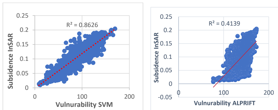
شکل ۶. نمودارهای ضریب همبستگی بین مدل‌ها و میزان فرونشست
