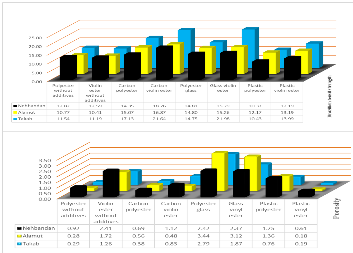
شکل ۷. نتایج آزمایش‌های تخلخل، ارتعاش فراصوت، کششی برزیلی و مقاومت بار نقطه‌ای نمونه سنگ‌های مصنوعی
