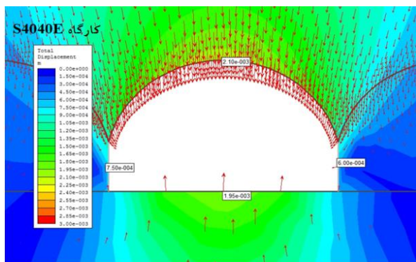
شکل ۵. مقطع کارگاه‌های استخراجی در بخش سولفور
