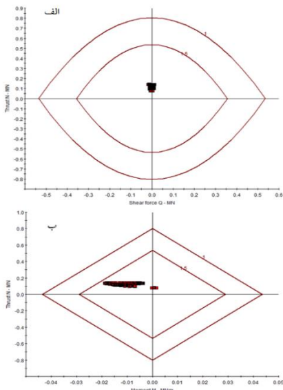
شکل ۲۰. نمودارهای الف: نیروی محوری-نیروی برشی و ب: نیروی محوری-گشتاور خمشی قاب فولادی با فاصله داری ۰/۸ متر.
