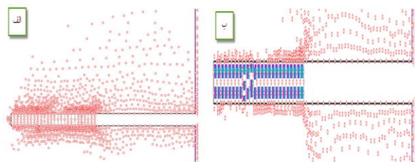
شکل ۲۶. ناحیه پلاستیک مقطع عرضی کارگاه S4058E الف: بدون سیستم نگهداری و ب: با سیستم نگهداری.
