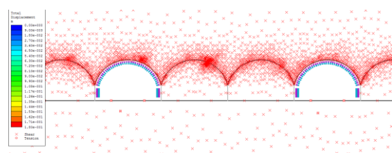
شکل ۱۸. زون پلاستیک ناشی از حفاری دو کارگاه با تاخیر در کانسنگ اکسیده تراز ۲۷۴۱.
