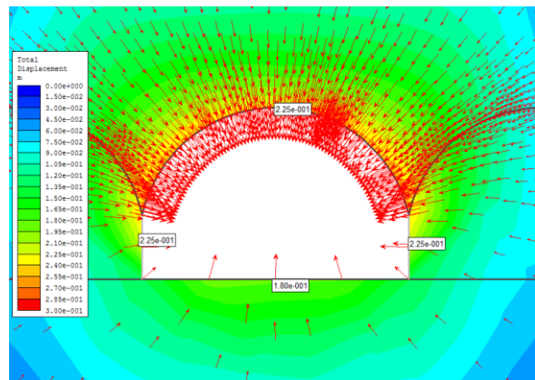
شکل ۱۰. کانتورها و بردارهای جابجایی اطراف یک کارگاه حفاری شده در کانسنگ اکسیده تراز ۲۷۴۱.
