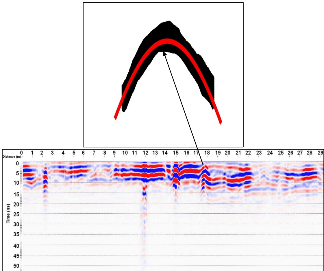
شکل ۷. هذلولی برازش یافته با الگوریتم PSO بر روی هذلولی پاسخ لوله انتقال فاضلاب در نگاشت راداری واقعی مربوط به پروفیل Pro1.
