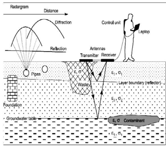
شکل ۲. الف) برداشت داده‌های GPR بر روی یک هدف مدفون و رخداد مربوطه در نگاشت راداری به صورت یک هذلولی (خط چین)، ب) نمایش بعضی از کاربردهای متداول GPR (Knödel et al., 2007; Daniels, 2004).
