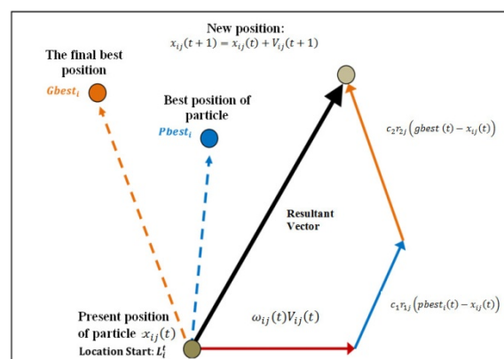
شکل ۵. نحوه تغییر موقعیت ذرات در الگوریتم PSO
