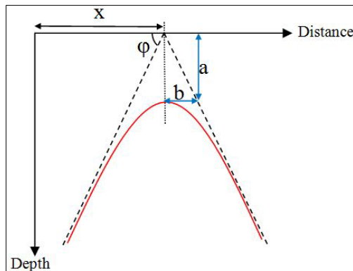
شکل ۴. پارامترهای هذلولی پاسخ GPR یک استوانه مدفون با شعاع معین در حوزه مکانی.
