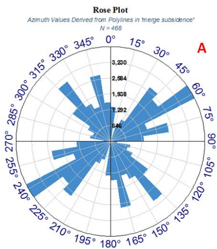
شکل ۱۰. نقشه‌های شکاف A: محدوده بشرو-جبلی، B: محدوده حسینی، C: محدوده کاریزک کنار کال، D: محدوده اردمه، E: محدوده کلاته قنبر
