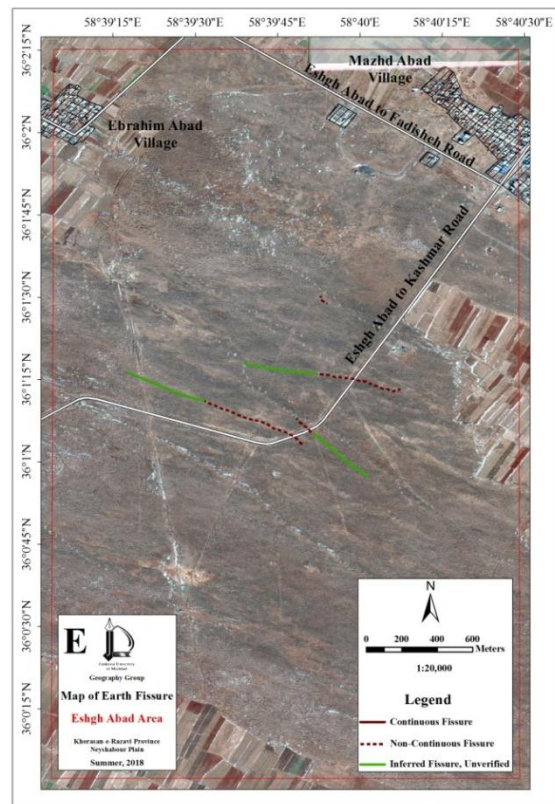
شکل ۹. نقشه‌های شکاف A: محدوده بازوبندی، B: محدوده تونزنده‌جان، C: محدوده کریم‌آباد، D: محدوده سلیمانی میان‌جلگه، E: محدوده عشق‌آباد
