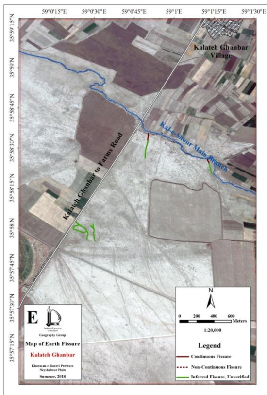
شکل ۱۰. نقشه‌های شکاف A: محدوده بشرو-جبلی، B: محدوده حسینی، C: محدوده کاریزک کنار کال، D: محدوده اردمه، E: محدوده کلاته قنبر
